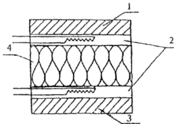
Рисунок А.1 - Схема прибора с одним тепломером
